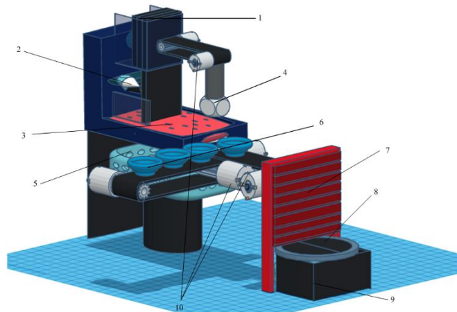
Рис. 1. 3D-модель годівниці «PetFeed»
